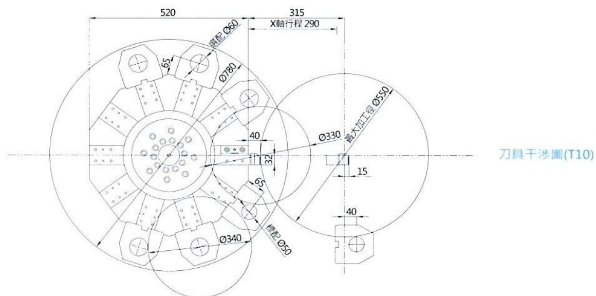
LA-350/LA-450 刀具干涉圖
